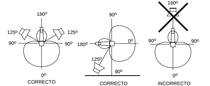
COLOCACION DE FUENTES SONORAS NO DESEADAS FIGURA 1
