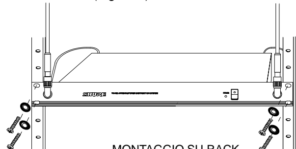
MONTAGGIO SU RACK FIGURA 6
