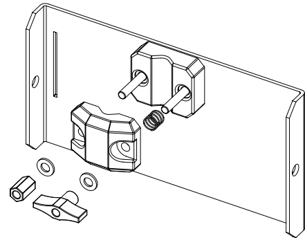
Abbildung 1: Auseinanderbau des WA596
