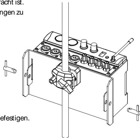
Abbildung 2: WA596 in zusammengebautem Zustand
