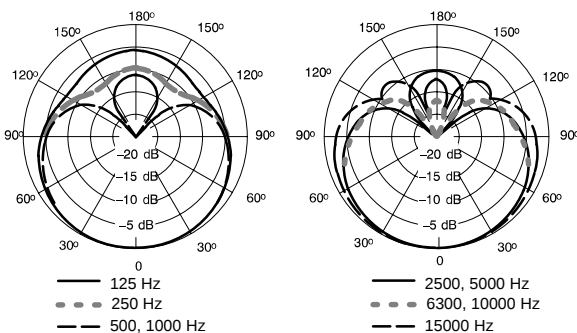
TYPISCHE RICHTCHARAKTERISTIK ABBILDUNG 3
