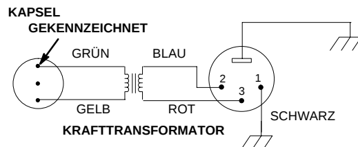
INTERNE SCHALTUNGEN ABBILDUNG 4
