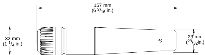
GESAMTABMESSUNGEN ABBILDUNG 5
