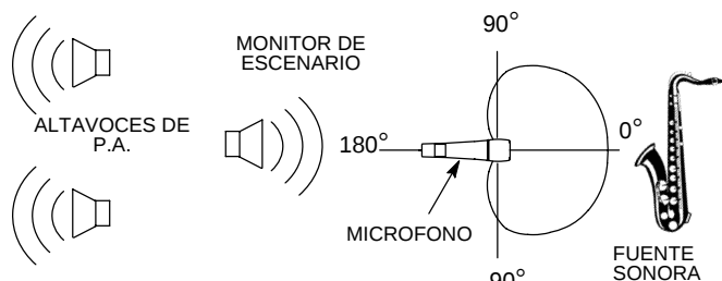
COLOCACION RECOMENDADA DE LOS ALTAVOCES
